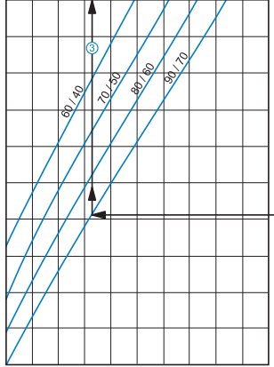
Temperatura powietrza po użyciu nagrzewnicy (°C) 5 10 15 20 25 30 35 40 45 50 55
