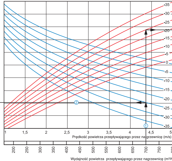
NKV 150-4 / NKV 160-4 / NKV 200-4
