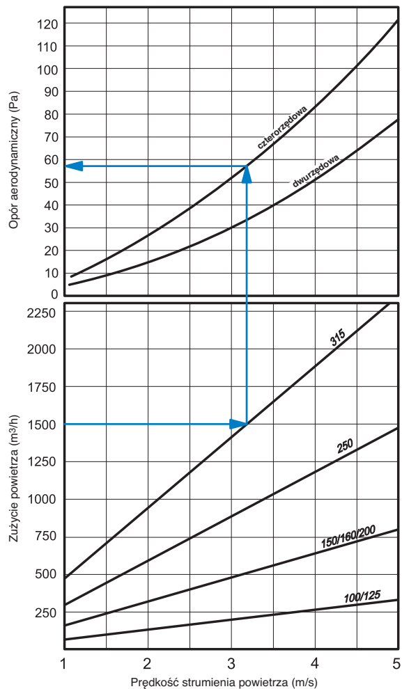
Strata ciśnienia powietrza nagrzewnic wodnych NKV
