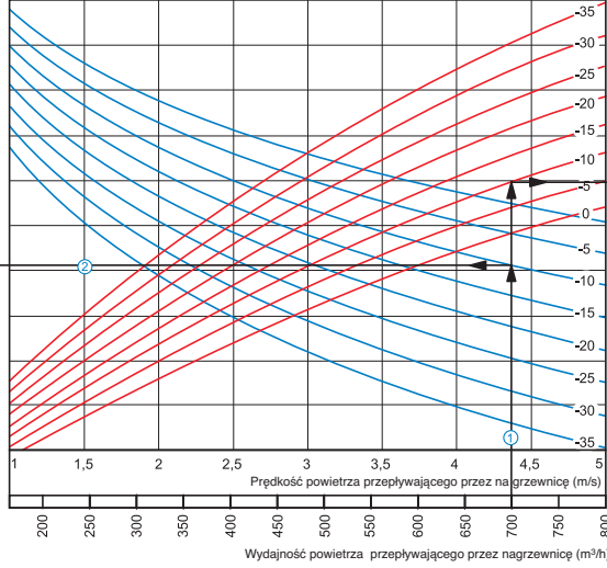
NKV 150-2 / NKV 160-2 / NKV 200-2
